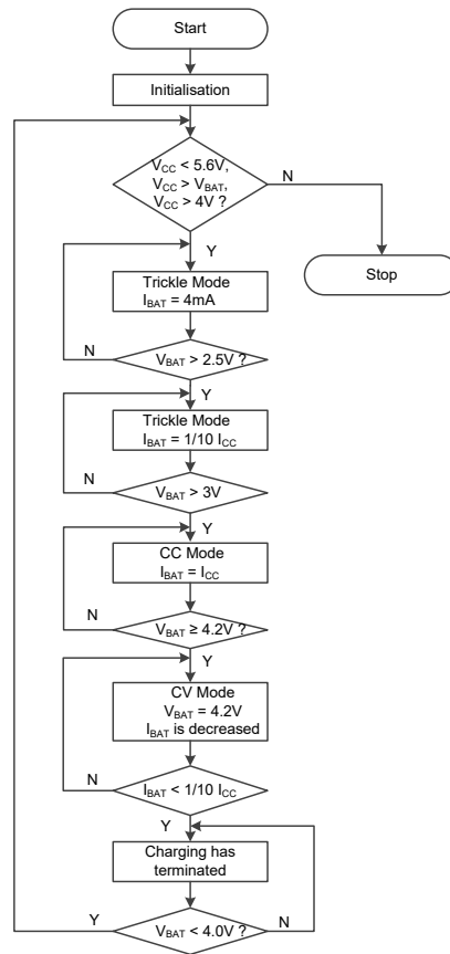
线性电池充电器流程图
